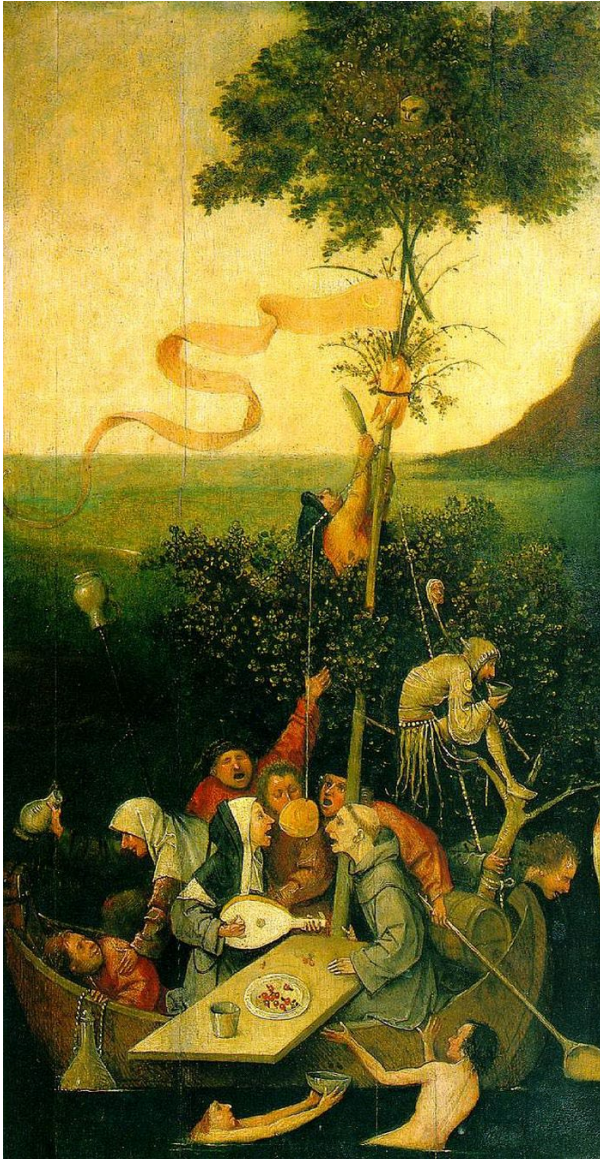
Het Narrenschip ca. 1494 of later Hiëronymus Bosch Olieverf op paneel 58 × 33 cm Louvre Parijs, Frankrijk
